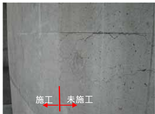
図-6 施工境界付近の状況
