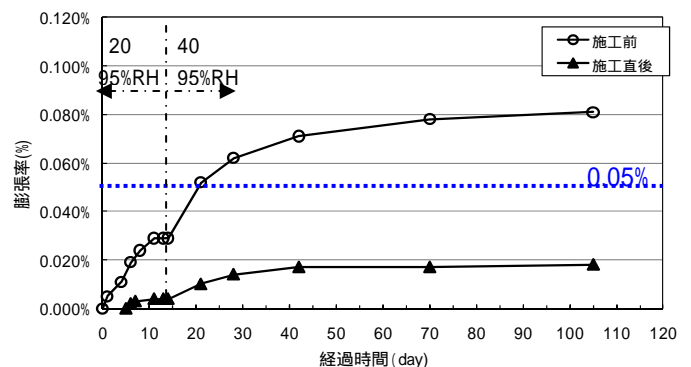
図-1 JCI-DD2 法による残存膨張量
