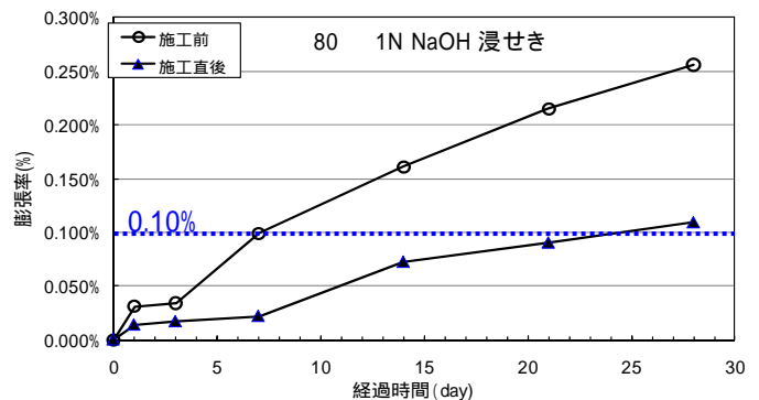
図-2 カナダ法による残存膨張量
